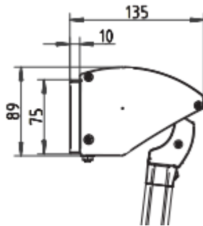
DA320 mål inkl. Vægbeslag
