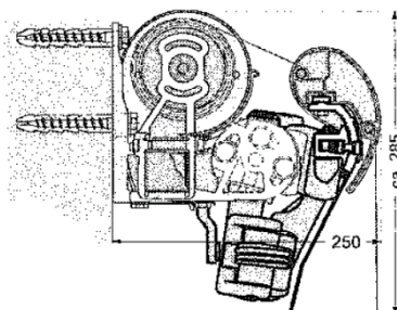
Design Krydsarm Basic mål inkl. vægbeslag
