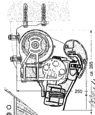
Design Krydsarm Basic mål inkl. loftbeslag
