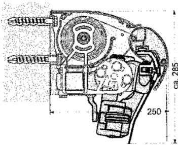
Design Krydsarm Super mål inkl. vægbeslag
